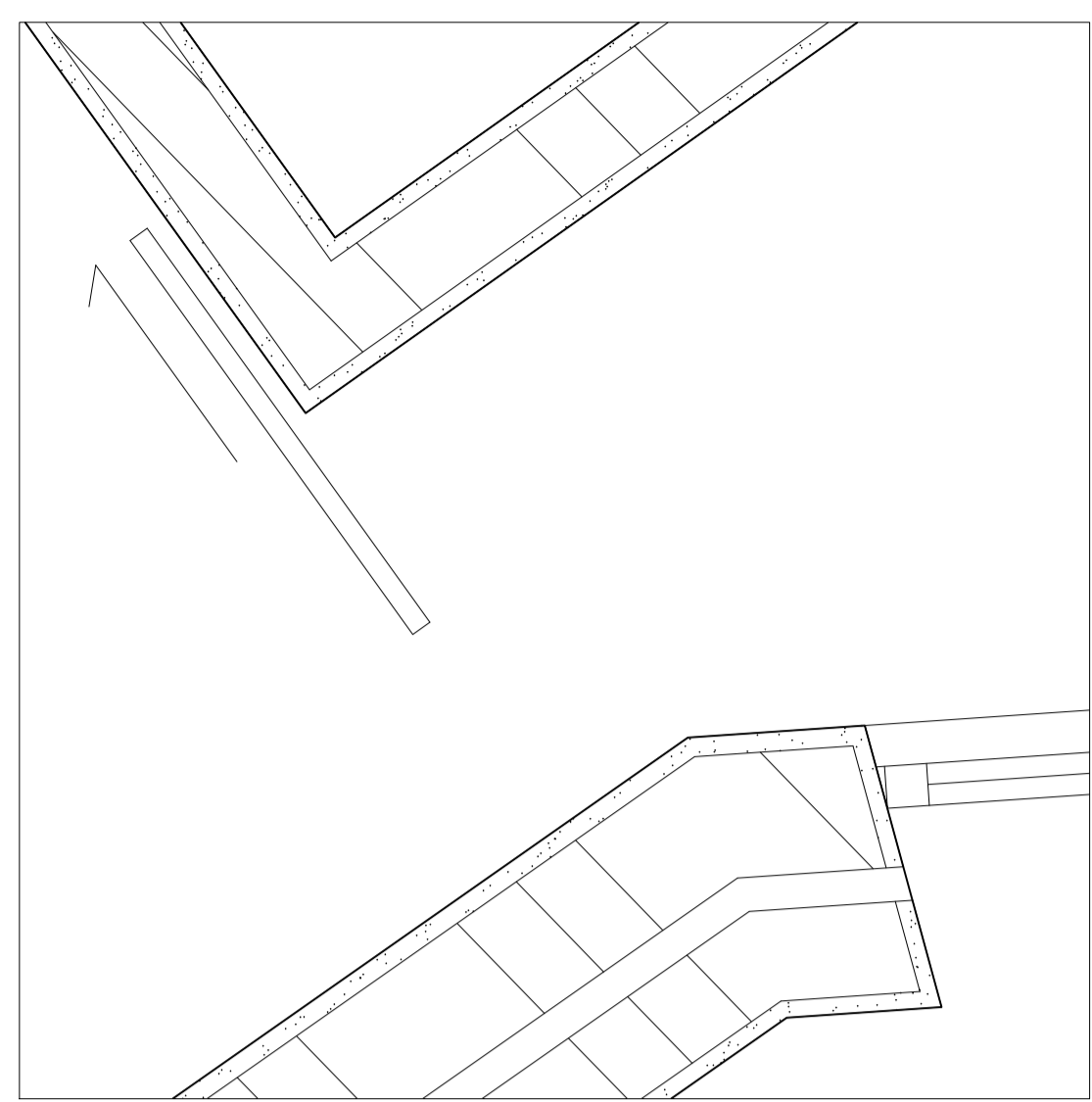
Pormenor da planta escala 1/20
