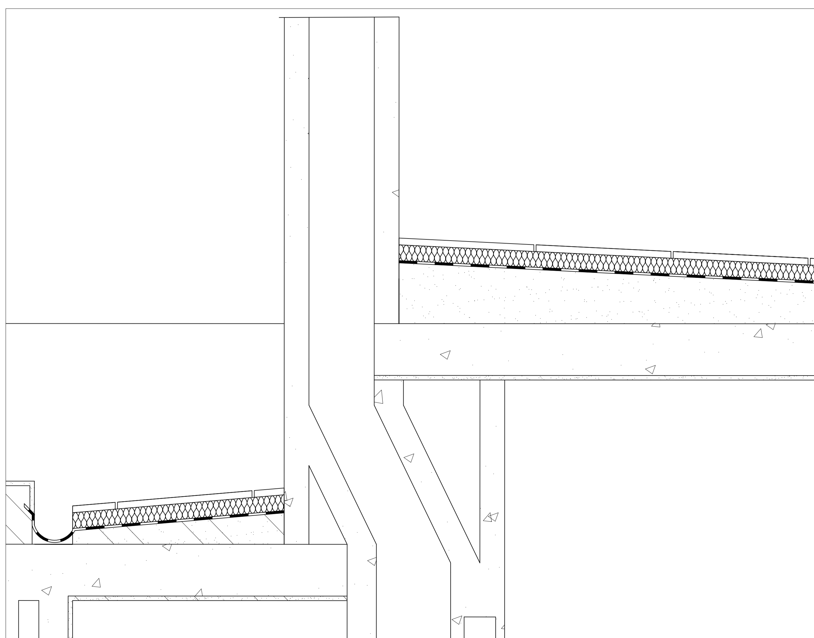
Pormenor do corte escala 1/10
