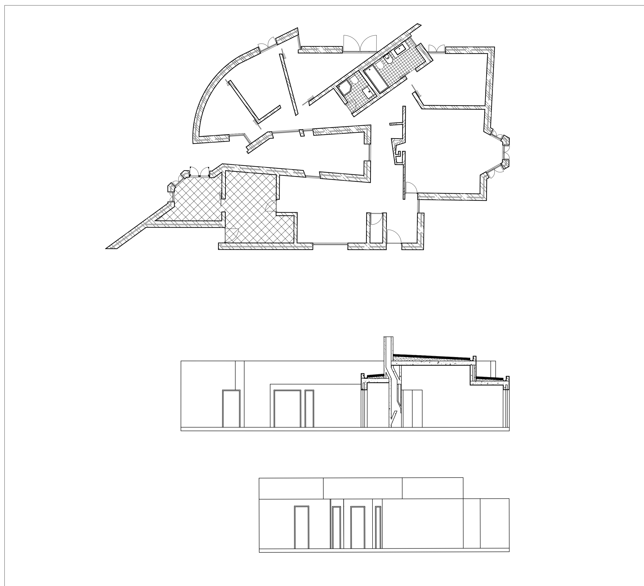
Planta, corte e alçado articulados escala 1/100
